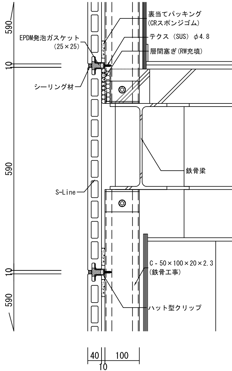
一般梁部断面詳細図
