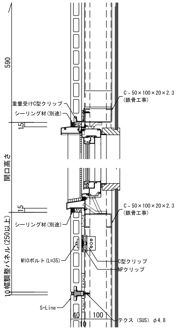
開口部断面詳細図
