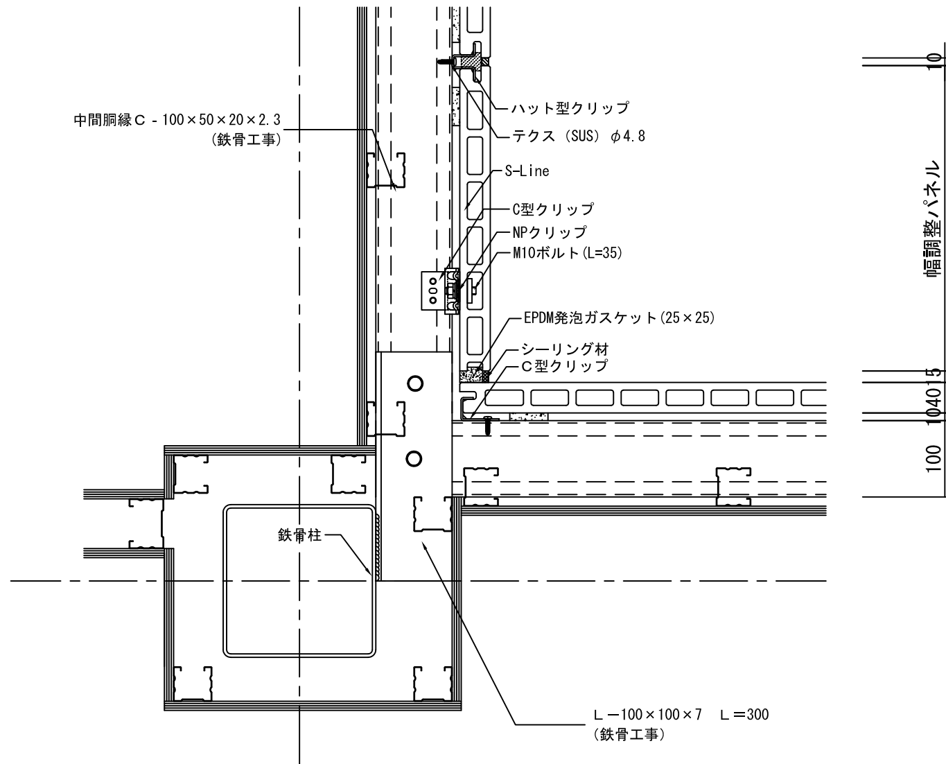
中間胴縁平面詳細図
