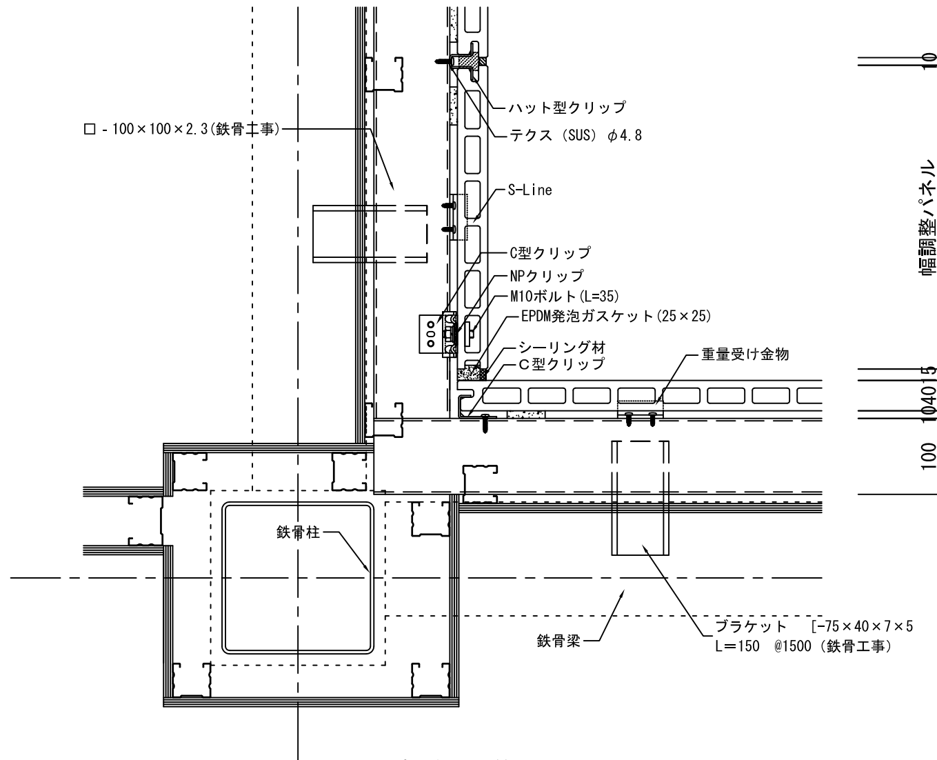
梁部胴縁平面詳細図
