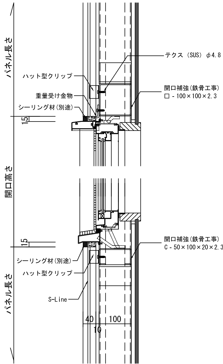
開口部断面詳細図
