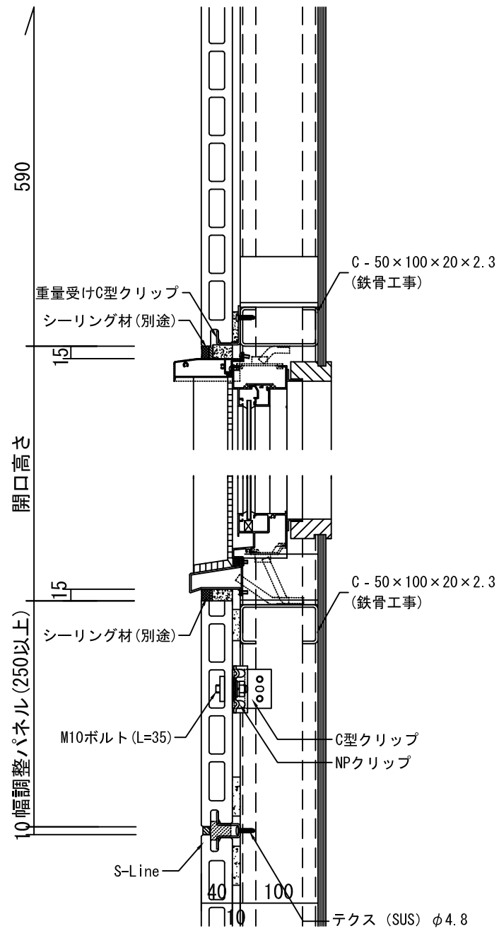
開口部断面詳細図
