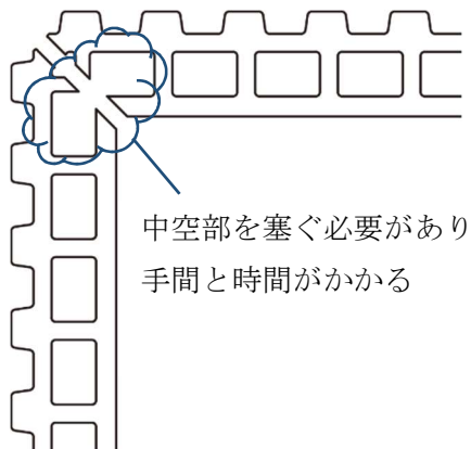
&lt;従来のタスロック45度切断コーナー&gt;
